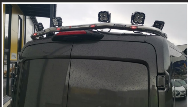
15054 Työvaloteline (H2 kattokorkeus)
